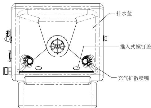
平面图（已移处盖）
