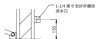
详图 C 比例尺 1:10
