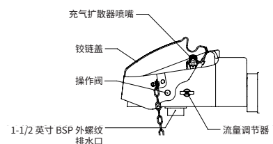
详图 B 比例尺 1:10
