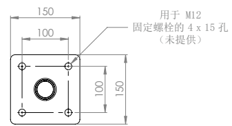
详图 A (固定细节) 比例尺 1:8
