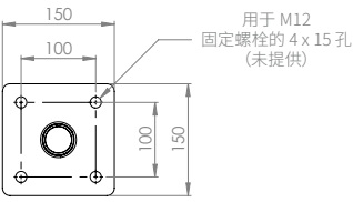
详图 A (固定细节) 比例尺 1:8
